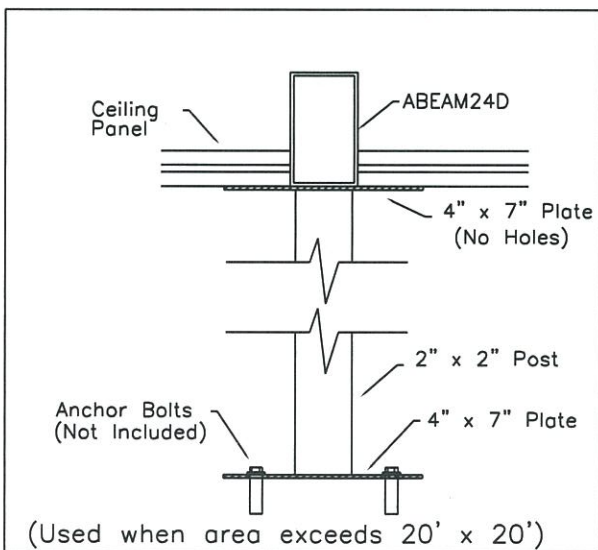
Support Post (JSC)
